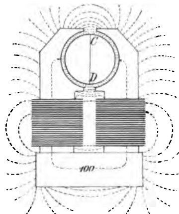
Abb. 139. Magnetische Streuung bei einer zweipoligen Gleichstrommaschine.
